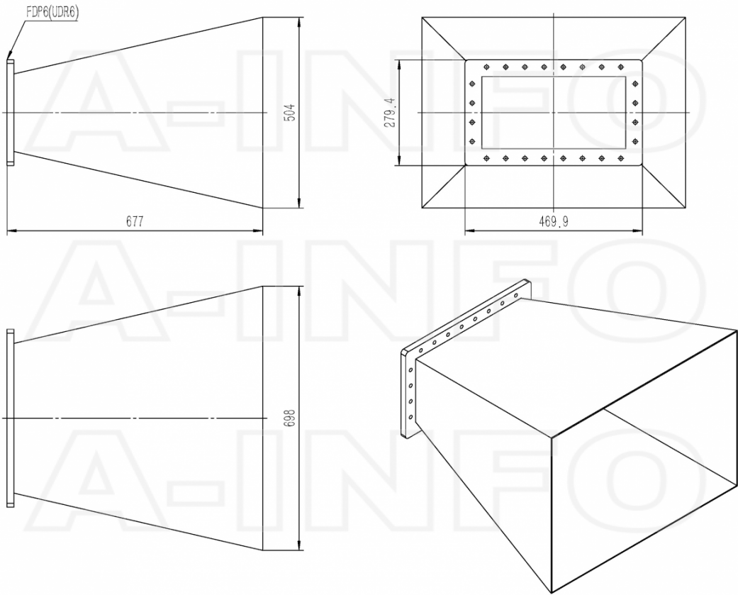
FDP6 Output (P/N: LB-1500-10-A)
